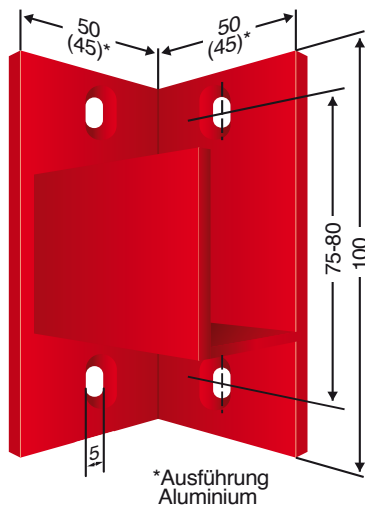
Balken-Halter
