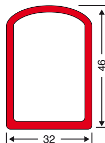
Balkenprofil
